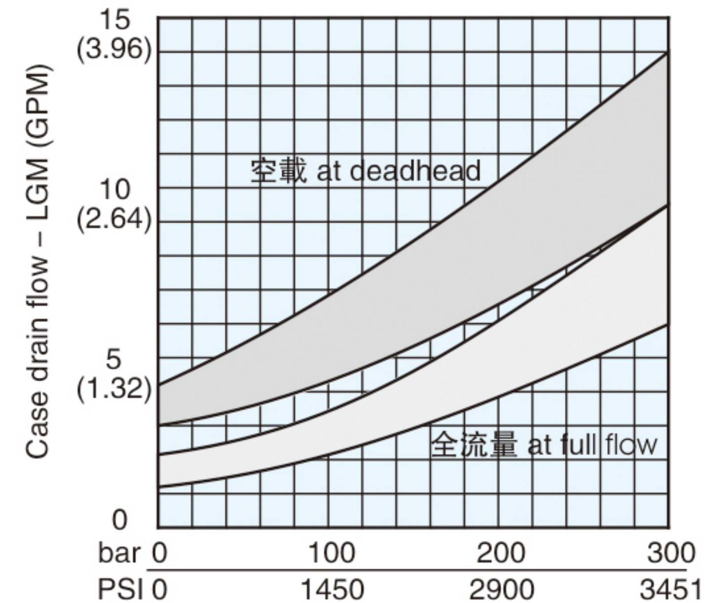
洩漏油特性PV140~PV180
