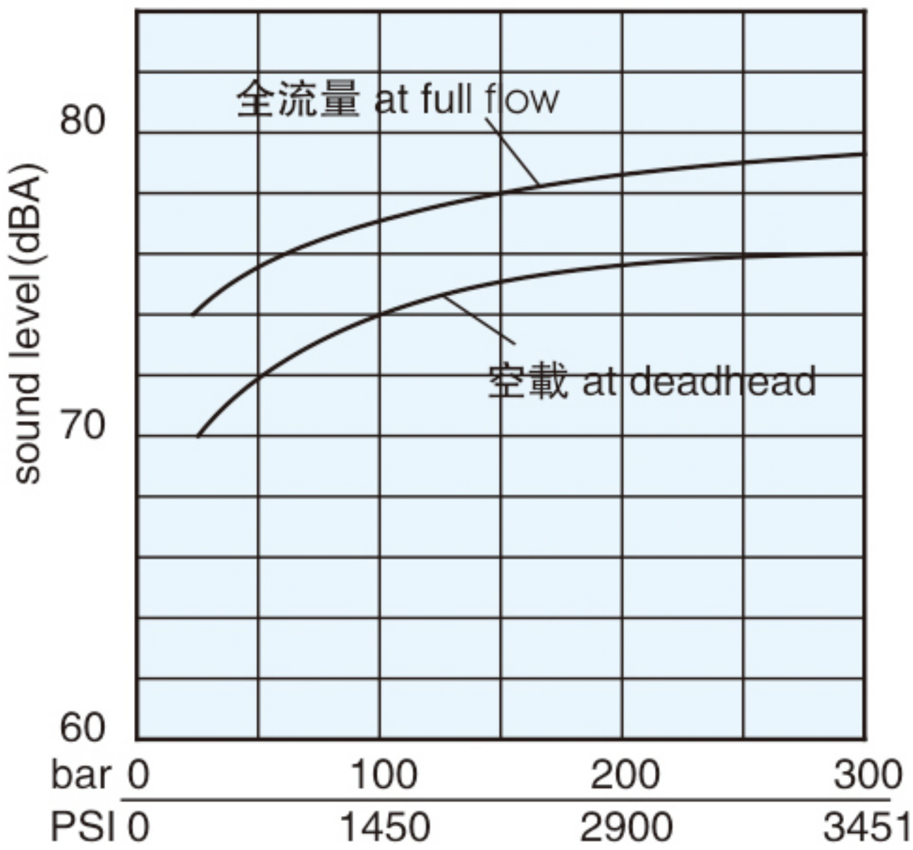
噪音級PV270
