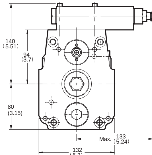
X向視圖 (View X)
