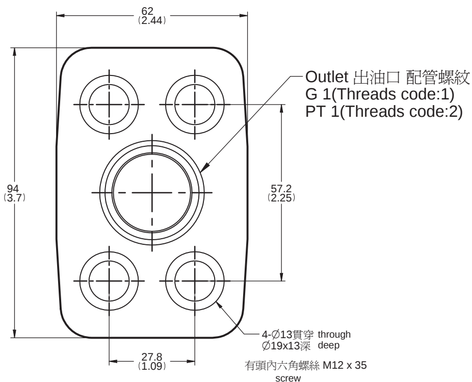
Outlet Flange 出油法蘭
