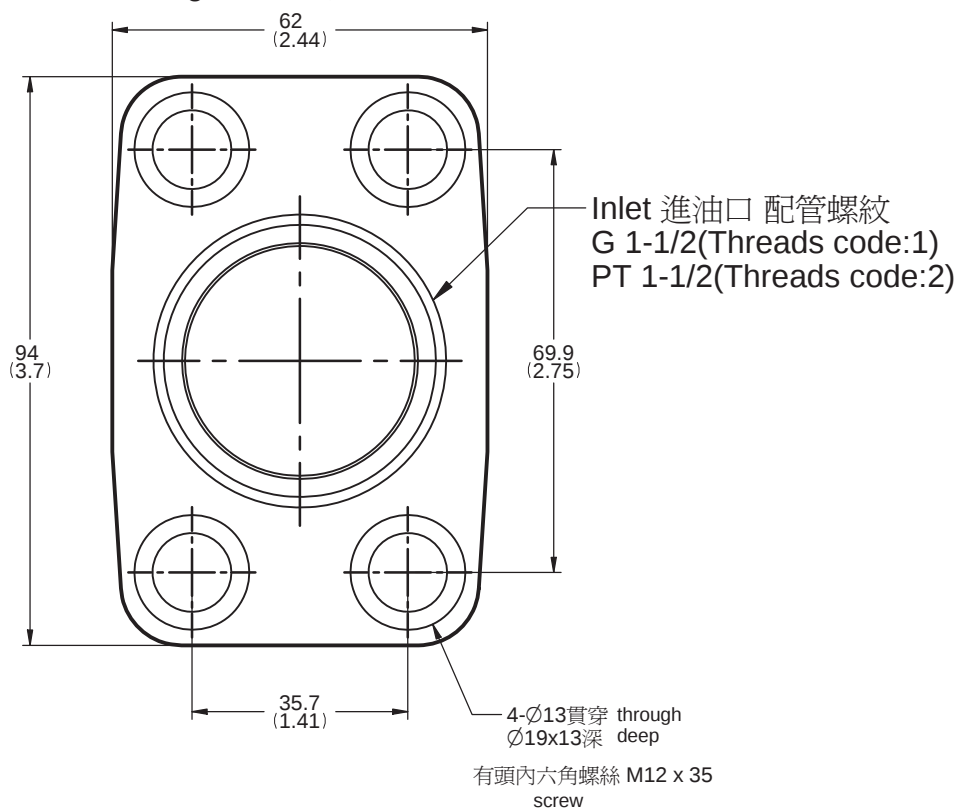
Inlet Flange 進油法蘭
