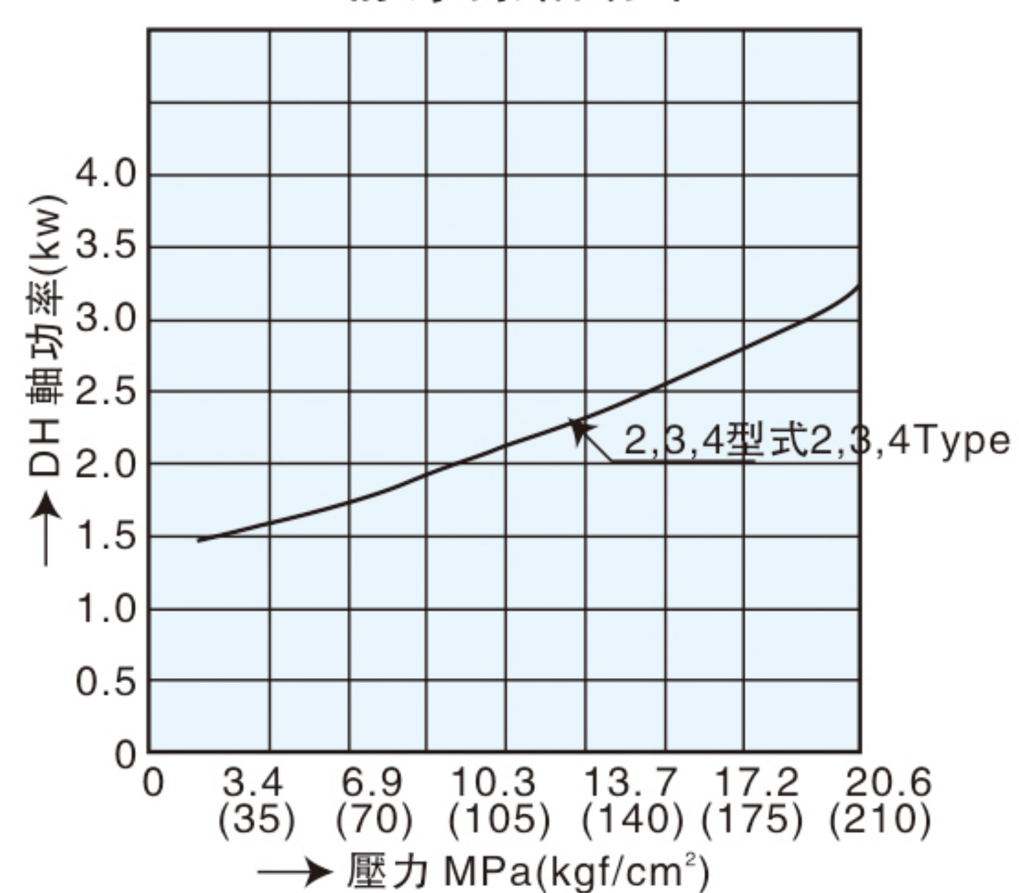
靜摩擦軸功率
