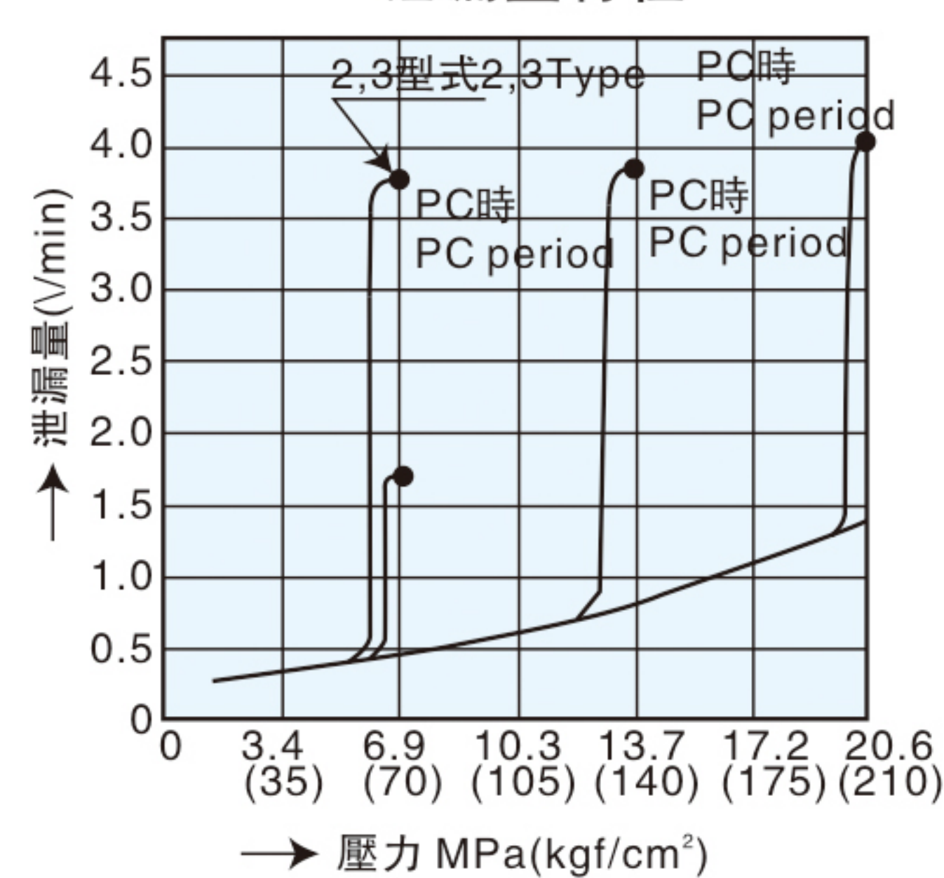
泄漏量特性
