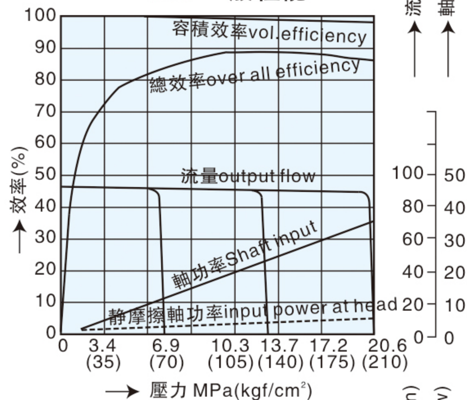
V70 一般性能
