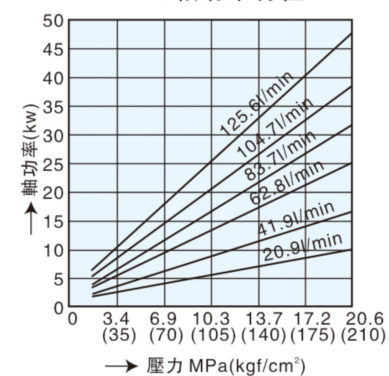
V70 軸功率特性
