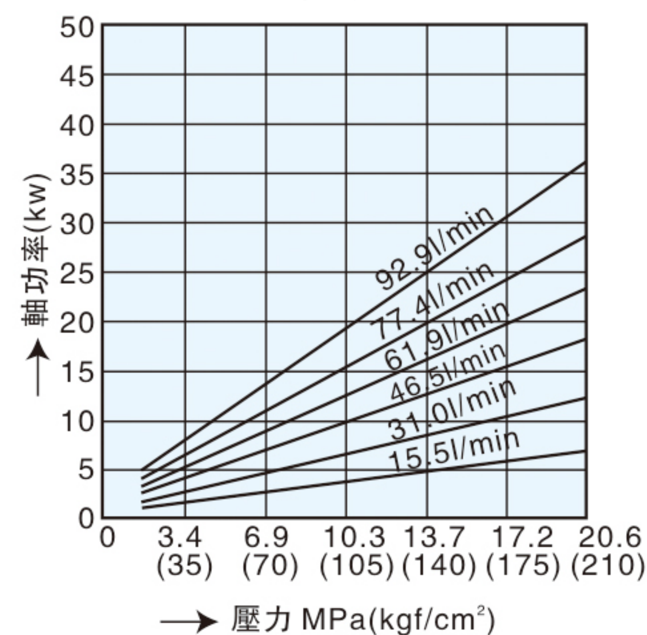
V70 軸功率特性
